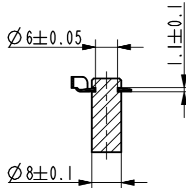
Einbausituation / assembly situation 1:1
